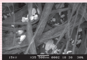
パイルの中に閉じ込めたダストの 電子顕微鏡写真
