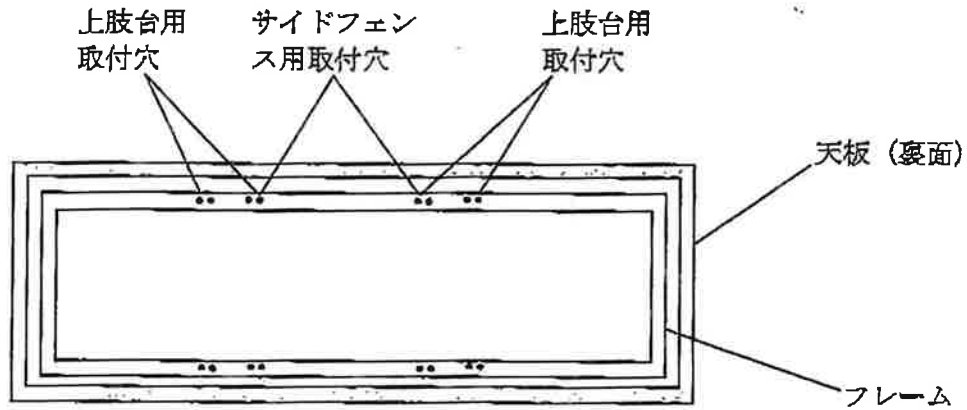
取付金具の取付方法
